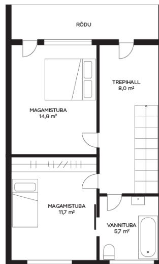
II KORRUS
